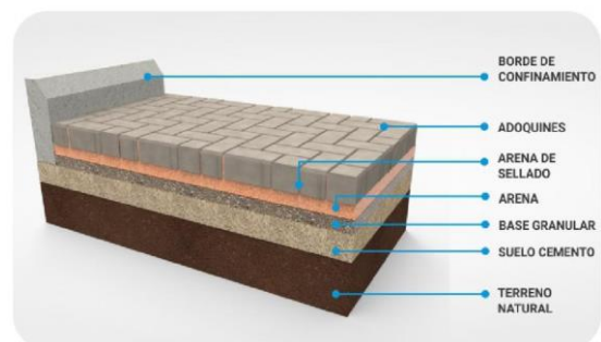
Detalle Arquitectónico
